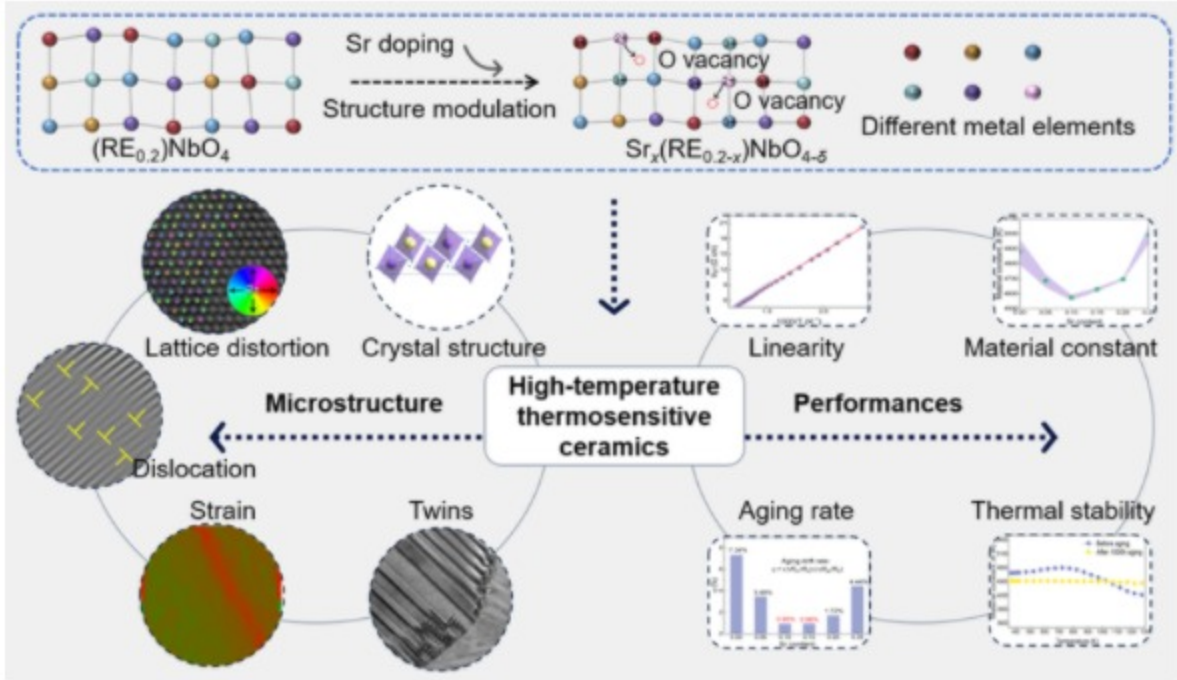
高温热敏陶瓷微观结构与性能关系
