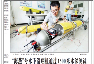
“海燕”号水下滑翔机通过1500米水深测试
