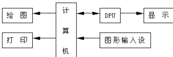
图 2-2-4 交互型绘图系统的硬件组成
