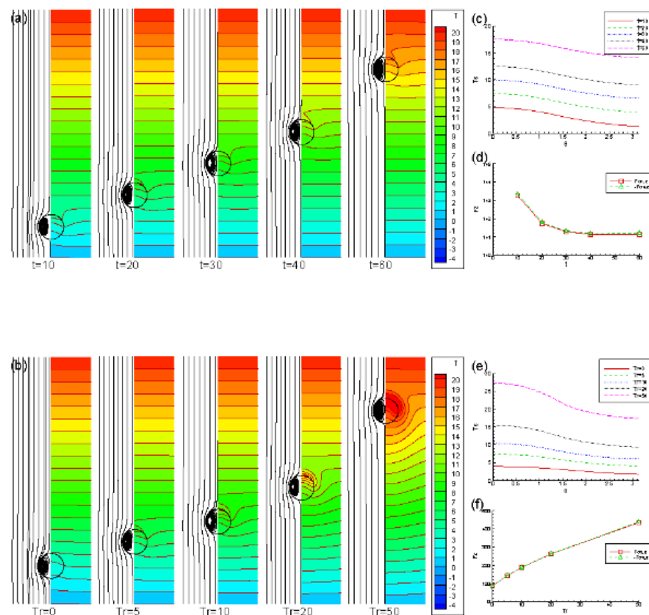
图: 随时间和热辐射数变化的液滴内外流场、温度场、界面温度分布和总的表面张力。
