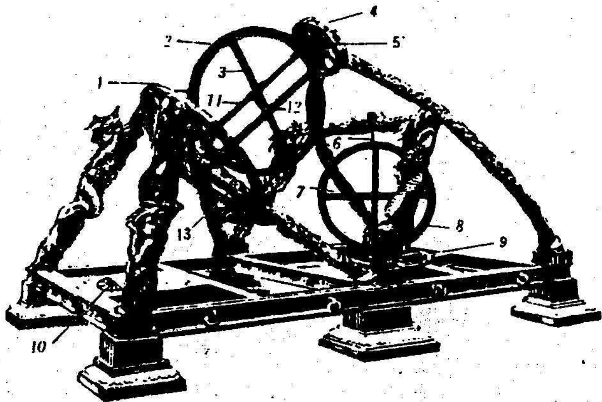
1—百刻环 2—四游双环 3—窥管 4—候极环 5—北极 6—天顶 7—地平 8—立运环 9—阴 纬环 10—日晷 11—直距 12—横关 13—界衡
