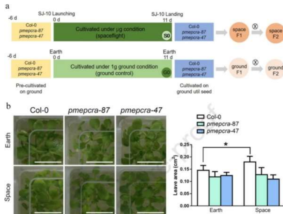
图1 拟南芥Col-0野生型与atpmepcra T-DNA插入突变体幼苗在微重力或重力生长条件下的平均叶面积比较
