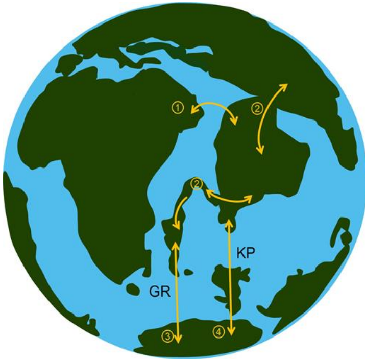
冈瓦纳古陆解体后 (88-55 Ma)，印度板块以及南极-澳大利亚-新几内亚板块与其他大陆之间可能存在的陆桥。(①非洲与印度的陆桥；②亚洲、印度、马达加斯加之间的陆桥；③南极-澳大利亚-新几内亚板块通过 Gunnerus Ridge (GR) 与印度板块相连；④南极-澳大利亚-新几内亚板块通过Kerguelen Plateau (KP) 与印度板块相连。) 地图改自Briggs (2003) 和Bossuyt et al. (2006)
