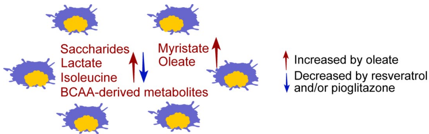
油酸暴露诱发的巨噬细胞胞外微环境代谢紊乱示意图
