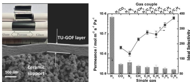
TU-GOF复合膜实物、截面形貌和气体渗透性能
