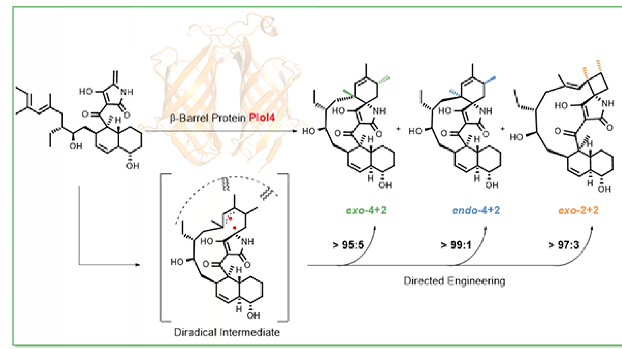
图 β-桶状蛋白催化的竞争性2+2/4+2环加成反应及基于选择性调控的定向进化
