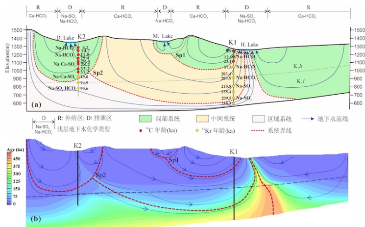
鄂尔多斯乌审召盆地地下水系统的多级嵌套结构：（a）图是地下水流系统多级嵌套结构示意图，（b）图是地下水流和年龄数值模拟结果。张俊 供图
