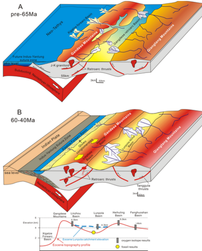
图3 重建青藏高原羌塘和拉萨地块印度和欧亚大陆碰撞前后升降模型
