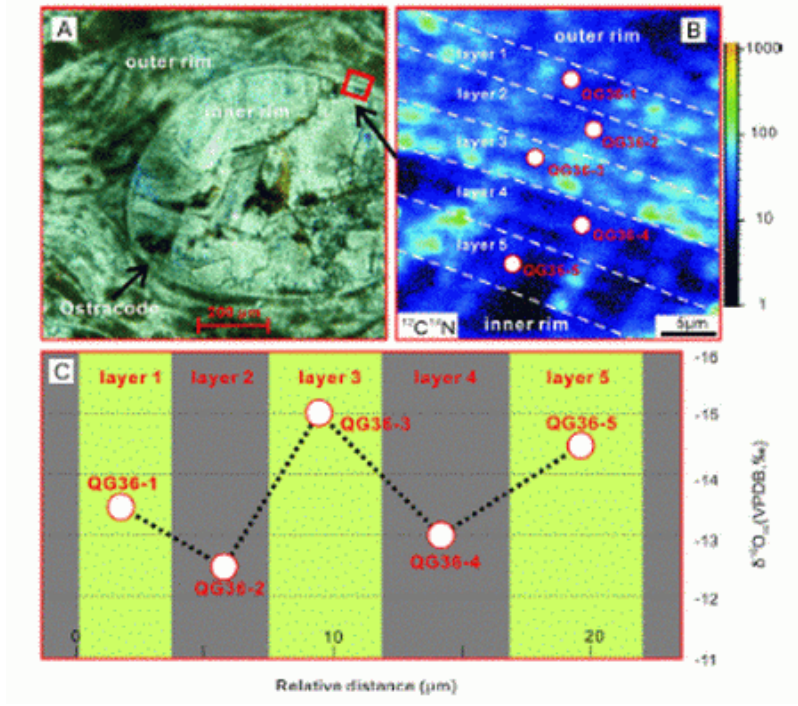
图2 介形虫化石壳体微区氧同位素变化特征，表明介形虫壳化石氧同位素没有受到后期成岩作用的影响。
