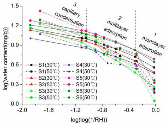
图2. FHH曲线确定吸附水状态界限
