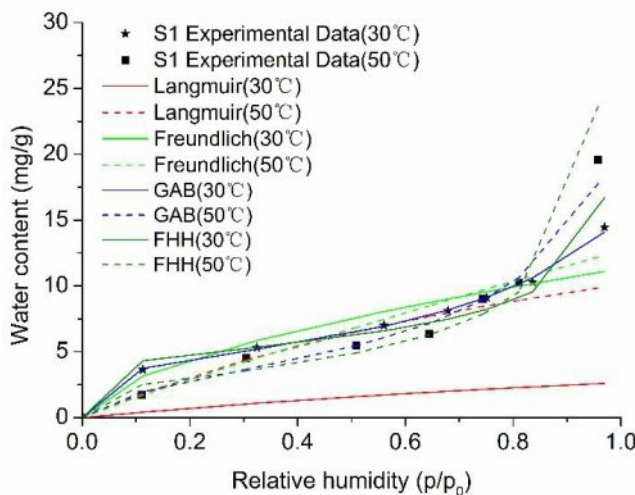
图1. 吸附模型与实验数据拟合
