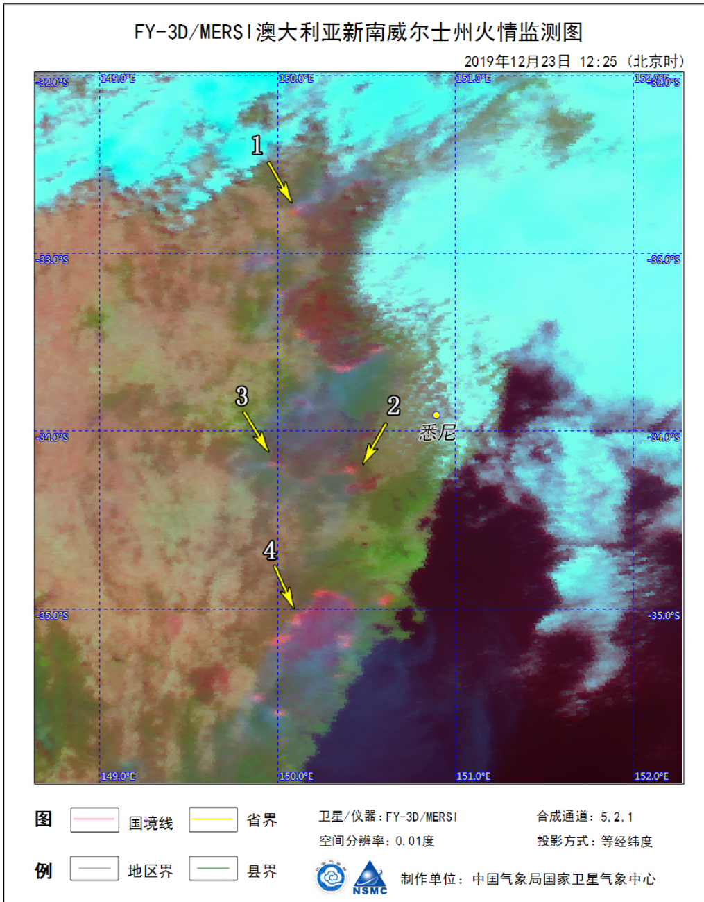
图为FY-3D气象卫星澳大利亚新南威尔士州火情监测图 2019年12月23日 12:25 (北京时间)
