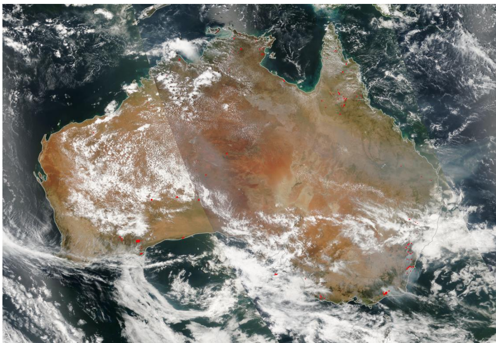
图为FY-3D/MERSI澳大利亚火情监测真彩色图（2019年12月23日）
