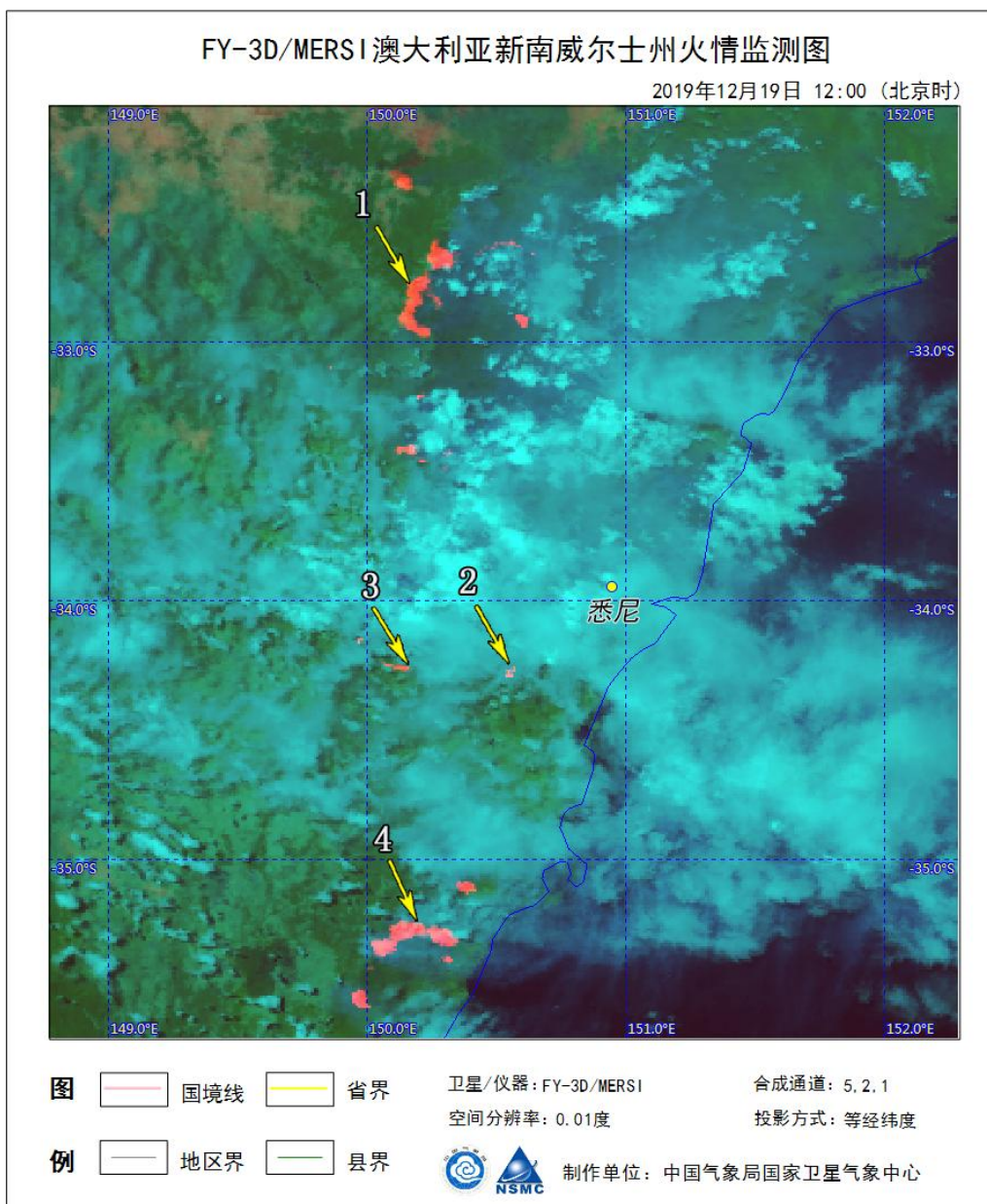
图为FY-3D气象卫星澳大利亚新南威尔士州火情监测图 2019年12月19日 12:00 (北京时间)
