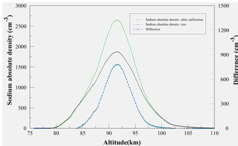
图二：钠层绝对数密度校正（Green）与原始（Black）比较
