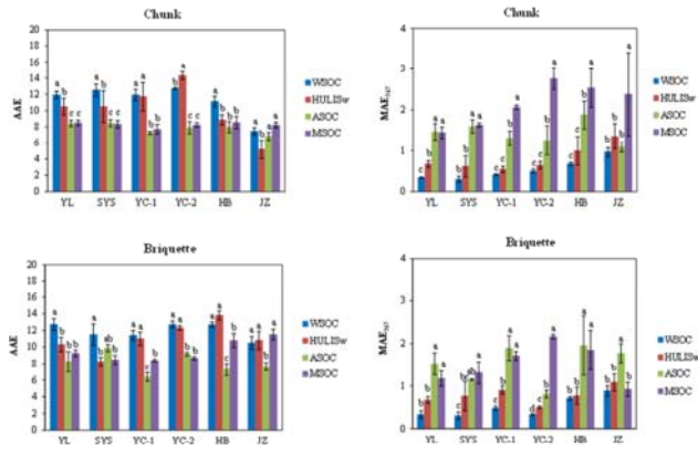
图1 不同类型燃煤排放BrC的Angstrom吸收指数(AAE)和光吸收效率(MAE365)
