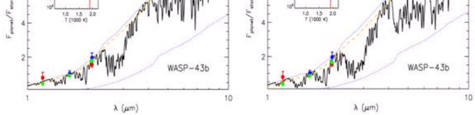
图2:行星与恒星亮度的比值图,其中蓝色点是该项工作的测量值,红色点是来自Gillon 等(2012)年的工作,绿色点是理论光谱换算成对应的测光数据的值。黑色曲线是理论光谱,其中左边图是假设太阳丰度比,右边假设金属丰度相对于太阳超丰5倍。小插图是行星大气的温度-压强轮廓。
