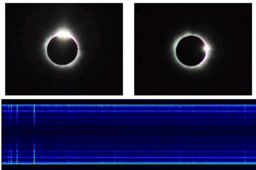
图1(上图)：日全食开始前后产生的贝利珠。图2(下图)：日食期间FASOT原理样机采集的积分视场单元内25个空间点产生具有相反偏振态的50条闪耀偏振光谱(50根光纤，从上到下)。从左到右第1、3和4条发射线为中性镁
