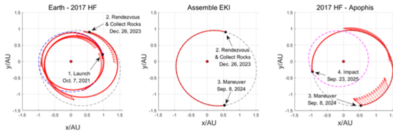
图三：“以石击石”全程轨迹优化
