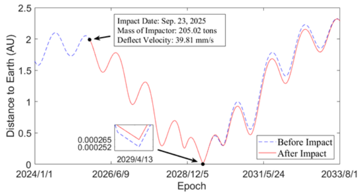
图四：撞击前后小行星相对地球的距离变化
