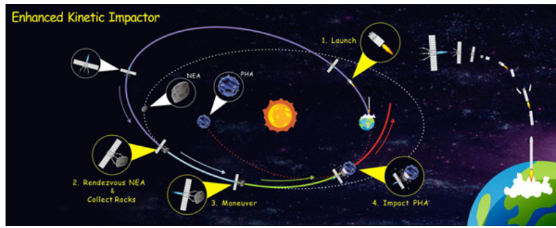
图二：“以石击石”行星防御任务方案示意
