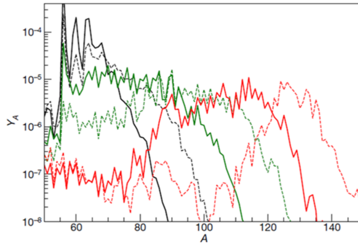
图1.在 Y_e=0.6 , \tau=10\text{ms} , S=80 (黑), 140 (绿), 200 (红) 的环境下, 实线代表增长的 3\alpha 反应率, 虚线是没有增长的, 可以看到核合成均被明显的压制, 重核素边界的质量数均被降低10到20 (金仕纶/图)
