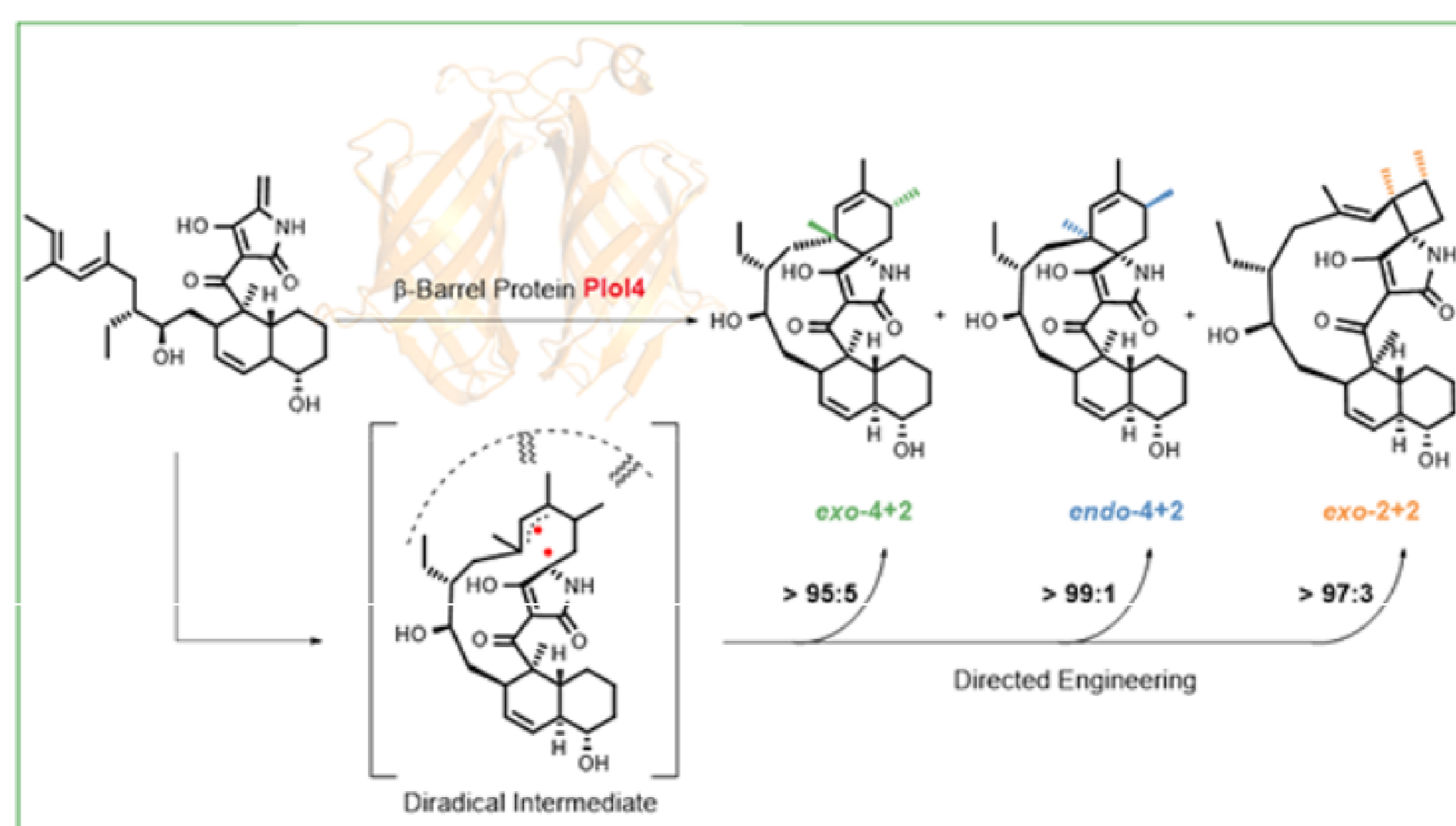
图 \beta -桶状蛋白催化的竞争性2+2/4+2环加成反应及基于选择性调控的定向进化
