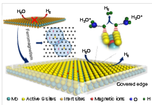
图1 长程铁磁性激活基面原子的示意图
