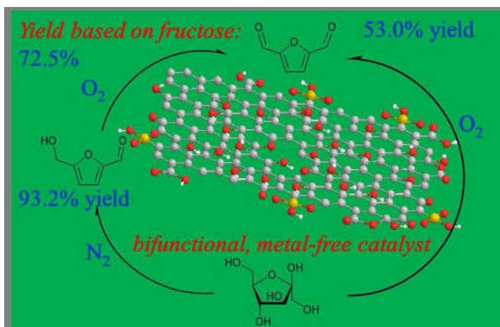
图2 非金属双功能氧化石墨烯催化果糖转化一步法制2,5-二甲酰基呋喃
