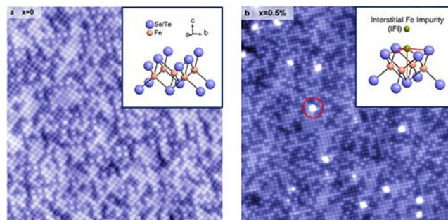
图1. \text{Fe}_{1-x}(\text{Te},\text{Se}) 样品中观测到的间隙铁杂质。
