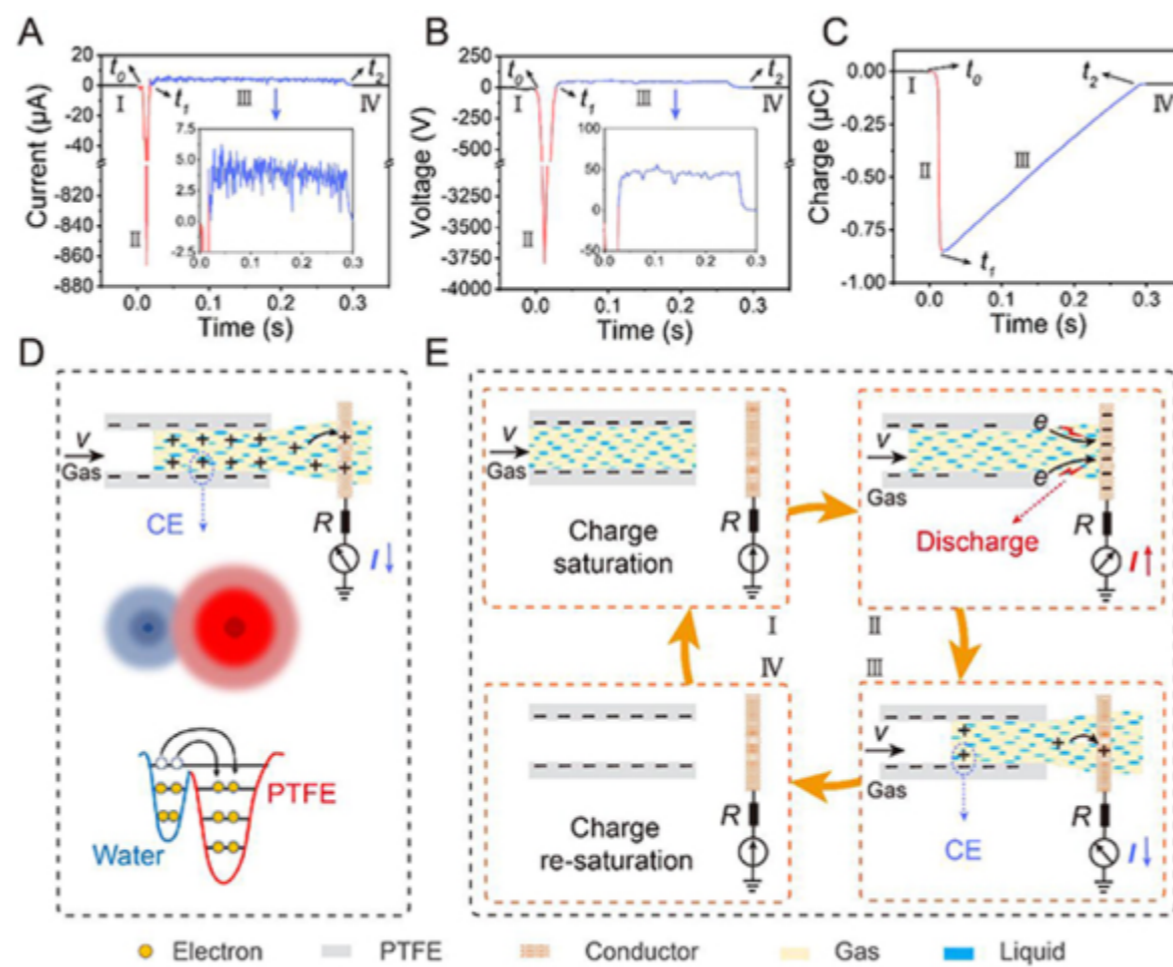
图3.气体-液体两相流摩擦起电机理研究示意图
