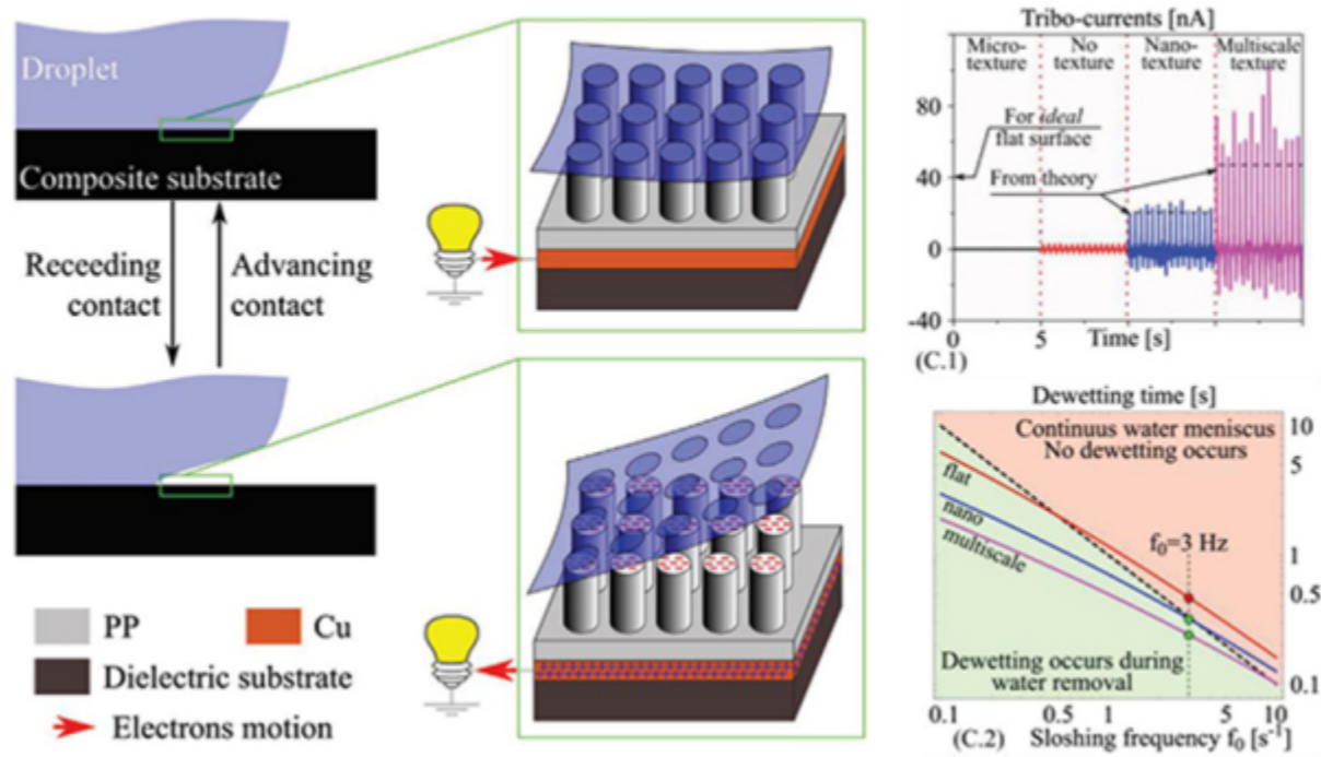
图2.固-液界面摩擦起电解析模型与润湿性转变跟踪
