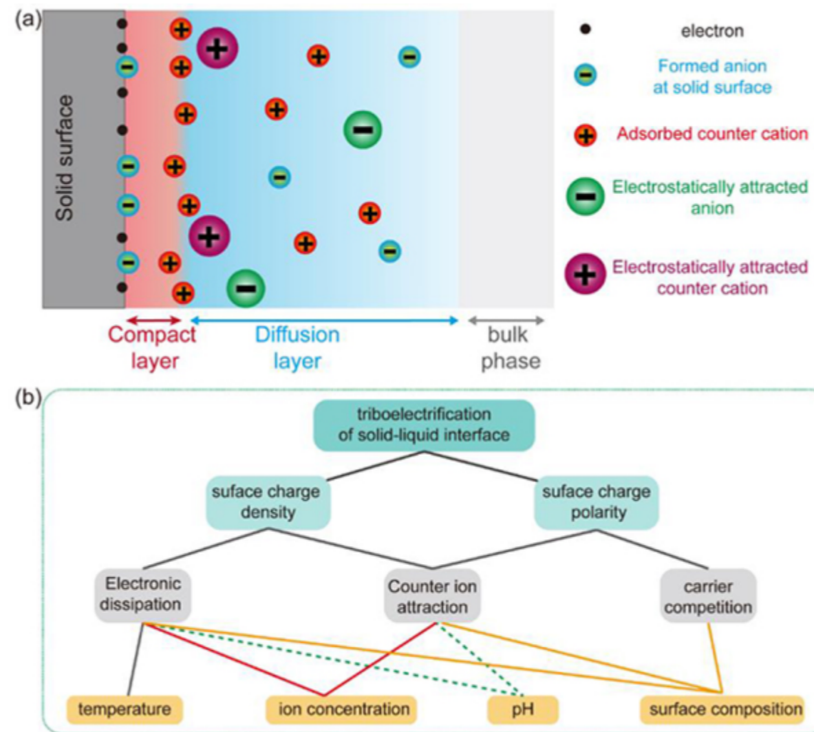
图1.固-液界面摩擦起电示意图及影响因素
