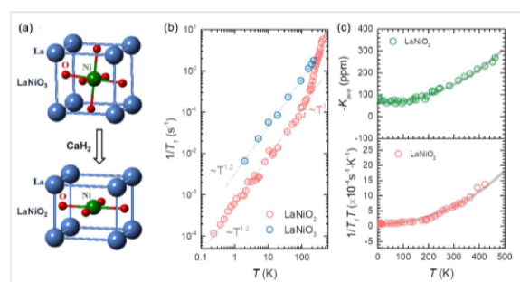
图: (a) LaNiO 3 和LaNiO 2 的晶体结构。通过CaH 2 还原LaNiO 3 可以得到LaNiO 2 。(b) LaNiO 2 和LaNiO 3 中自旋-晶格弛豫率 ( 1/T_1 ) 随温度的变化关系。(c) 上半图: LaNiO 2 的奈特位移 ( K_S ) 随温度变化的关系。下半图: LaNiO 2 中 1/T_1 随温度变化的曲线。
