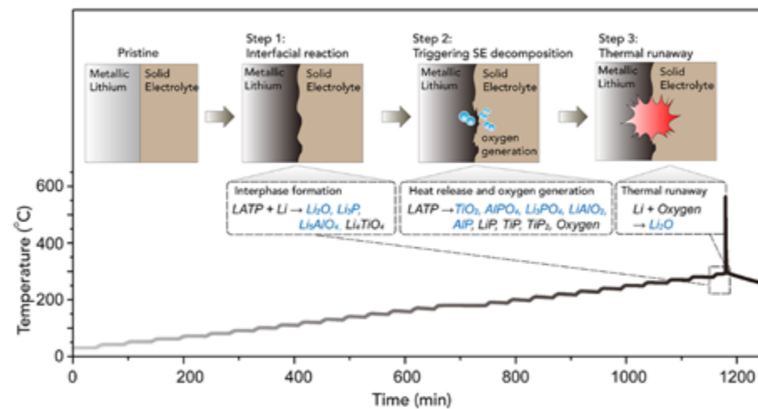
图3. 以LATP为例示意氧化物固态电解质-金属锂热失控反应机理。
