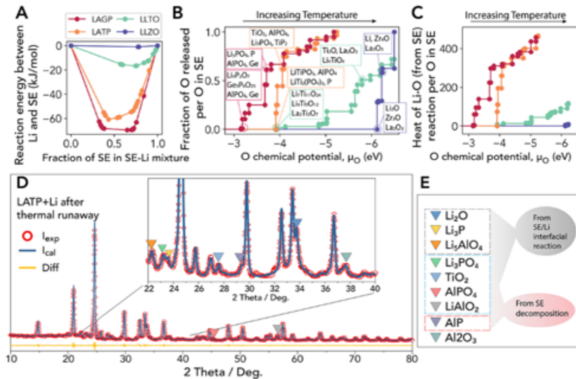
图2. a) 不同混合比例的氧化物固态电解质与金属锂反应的化学反应能；b) 氧化物固态电解质分解产生氧的难易程度对比；c) 氧化物固态电解质中氧与锂反应的放热量对比；d) LATP/Li热失控后残余样品的物相分析；e) XRD中各物相对应于固态电解质/锂界面化学反应产物和固态电解质分解产物的归属。
