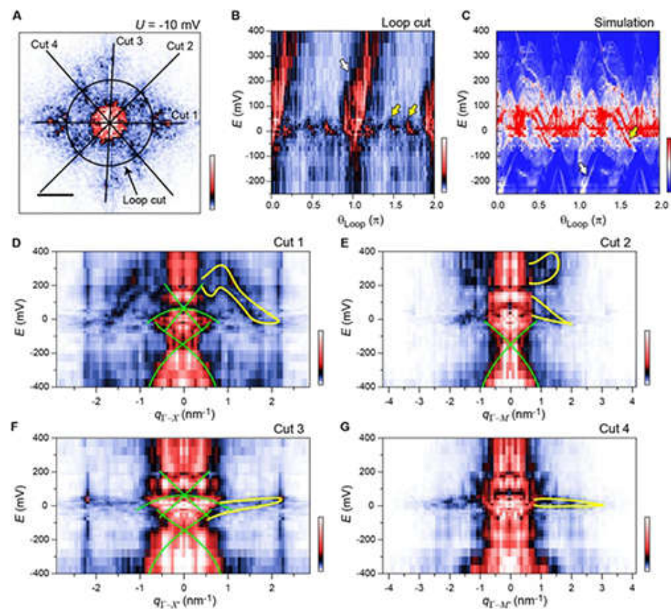
图2. 手性费米弧表面态的能量色散关系。(A) 实验获得的001面的准粒子干涉图案 ( E = -10 meV) ; (B) 表面态沿着A中黑色环线所切的能量E与散射波矢q的色散关系; (C) 与(B) 对应的计算模拟结果; (D-G) 沿着A中切线1到4所切得的E和q的色散关系
