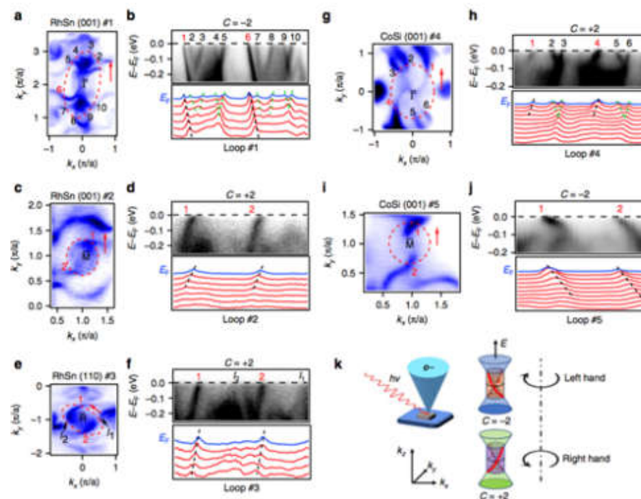
图4. ARPES测量显示CoSi和RhSn的螺旋型表面态能带具有相反的手性
