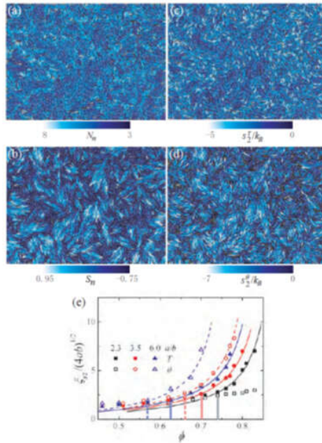
图二：胶体椭球系统中粒子的局域空间平移序分布（a）、角度序分布（b）、平移构型熵分布（c）和角度构型熵分布（d），以及各自空间关联尺度随密度的幂指数增大（e）。
