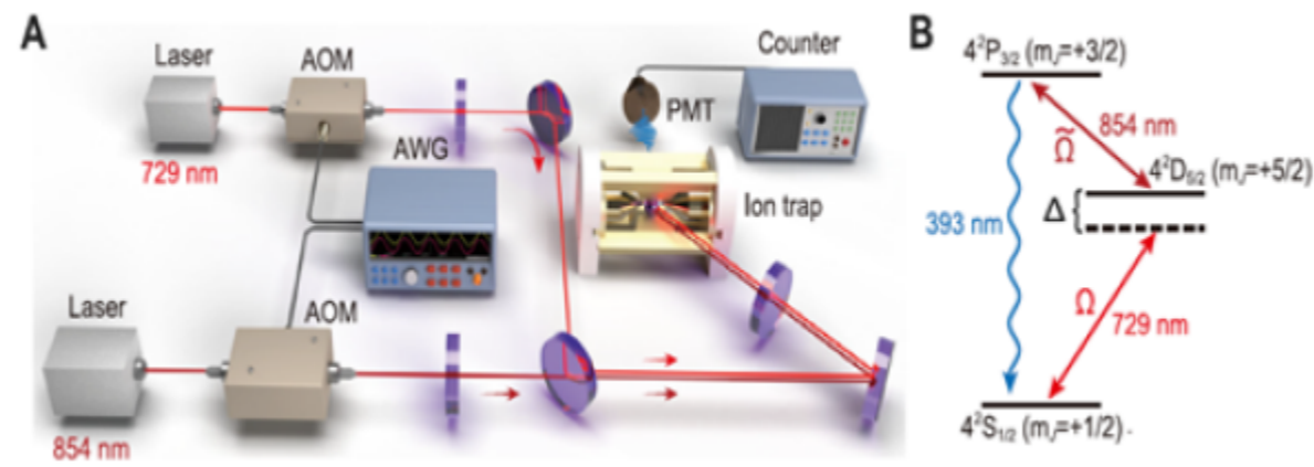
(A) 实验平台示意图，单个 ^{40}\text{Ca}^+ 离子在激光的精准操控下展现奥托热机的量子特性。(B) ^{40}\text{Ca}^+ 离子的能级示意图。
