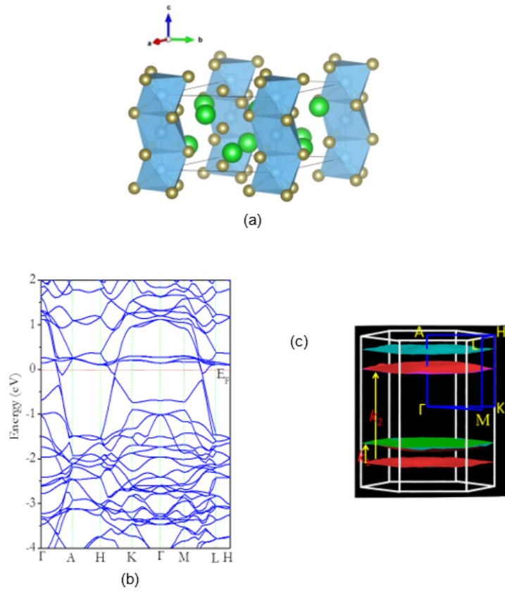
图1: \text{Ba}_3\text{TiTe}_5 的晶体结构(a)、常压能带结构(b)及费米面(c)。其晶体结构中含有沿c方向的共面八面体 \text{TiTe}_6 链, \text{TiTe}_6 链位于ab面内三角格点上, 在三角格子的中心有一个Te原子链。 \text{TiTe}_6 链和Te原子链由 \text{Ba}^{2+} 离子隔开, 形成一维导体。
