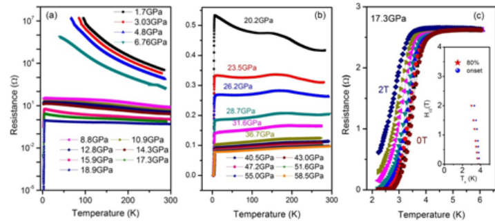
图2: 压力调控准一维材料 \text{Ba}_3\text{TiTe}_5 的磁电特性演化。(a) 在0-18.9 GPa压力范围的电阻随压力变化: 在较低压力由于倒逆散射效应材料呈现半导体行为; 在6.7-8.8 GPa压力区间, 低温电阻数据间突然下降5个数量级, 表明倒逆散射效应对电子输运行为的影响被抑制, 一维金属开始向三维金属过渡; 同时在8.8 GPa压力点观察到超导迹象。(b) 在20.2-58.5 GPa压力范围的电阻随压力变化: 除了超导现象之外, 在低温还发生了金属~半导体转变, 对应于SDW/CDW的产生; 同时在36.7 GPa压力附近观察到低温线性电阻行为, 对应于SDW/CDW被抑制后的量子临界点。(c) 在17.3 GPa压力, 超导转变随磁场方向的演化, 由此可以估算临界场。
