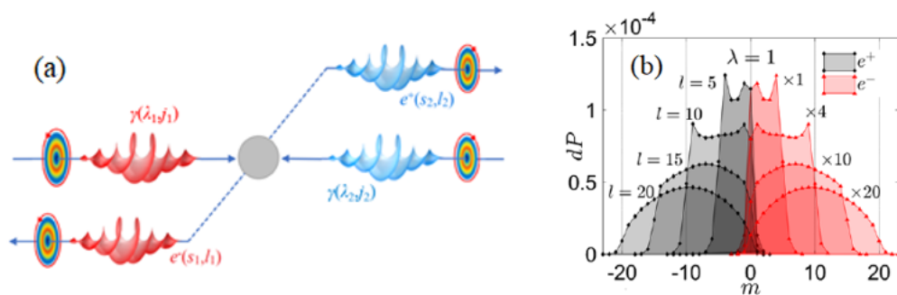
图1 (a)量子涡旋散射示意图. (b) Beth-Heitler过程产生的电子和正电子轨道角动量谱
