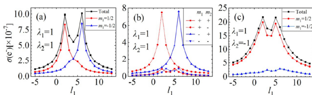
图2 Breit-Wheeler过程产生的电子在不同自旋下的轨道角动量谱. (a)、(b)和(c)分别对应不同的光子自旋极化
