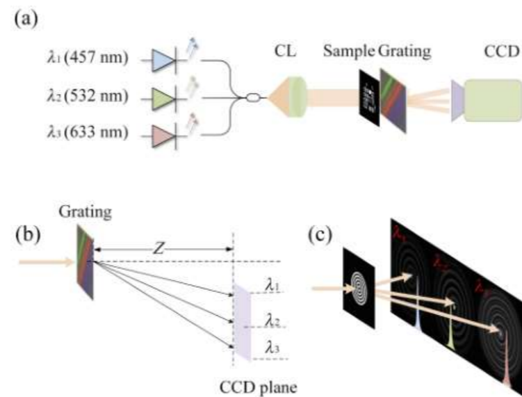
图1 多色光纤束单次成像光路
