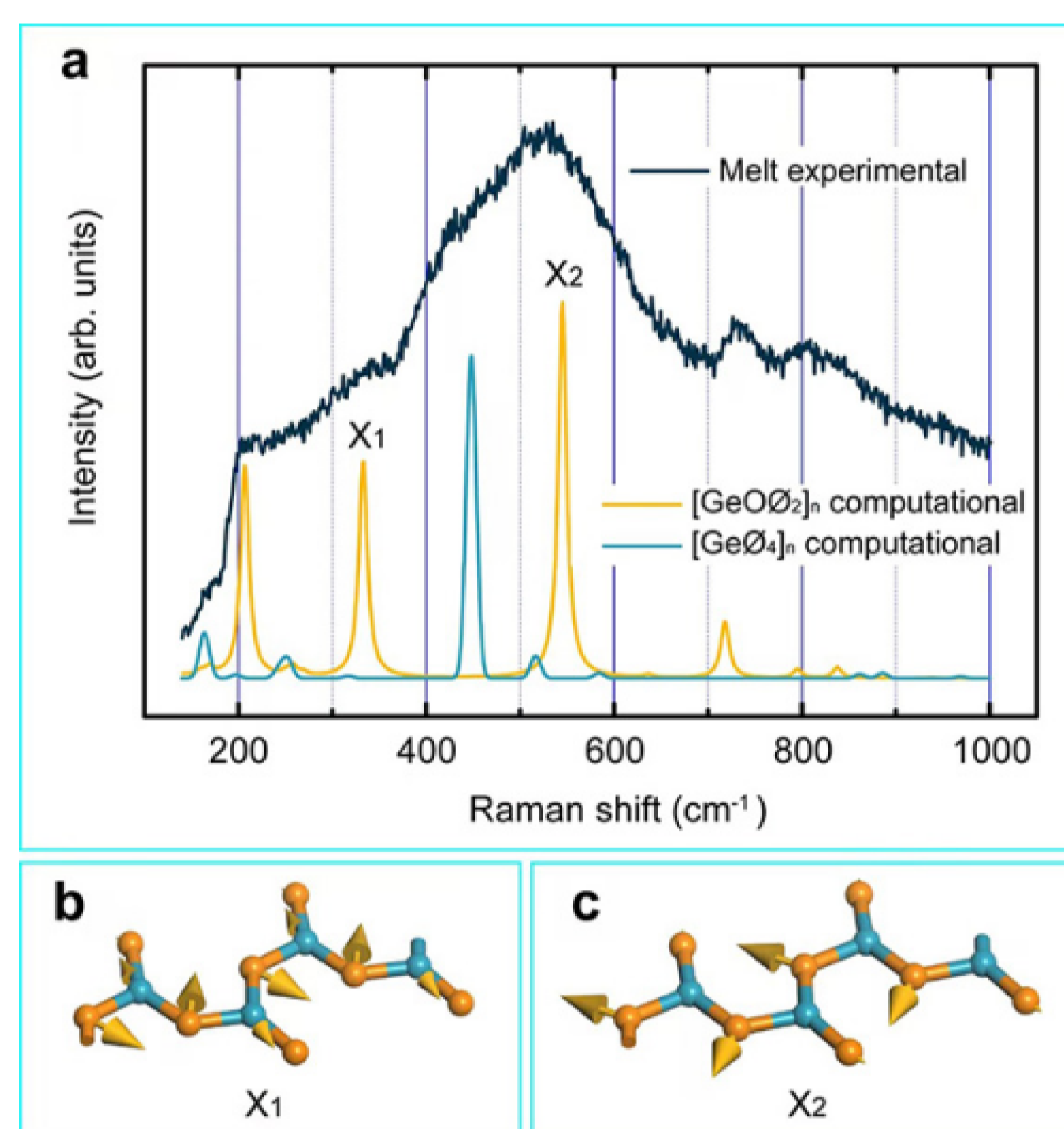
图1. \text{GeO}_2 熔体的拉曼光谱和两个特殊振动峰的振动模式。(a) \text{GeO}_2 熔体 (由 [\text{GeO}_2]_n 链和 [\text{GeO}_4]_n 网络构成) 的实验和计算拉曼光谱；(b) 340 \text{cm}^{-1} 拉曼峰的振动模式；(c) 520 \text{cm}^{-1} 拉曼峰的振动模式。蓝色和橙色小球分别代表锗原子和氧原子。
