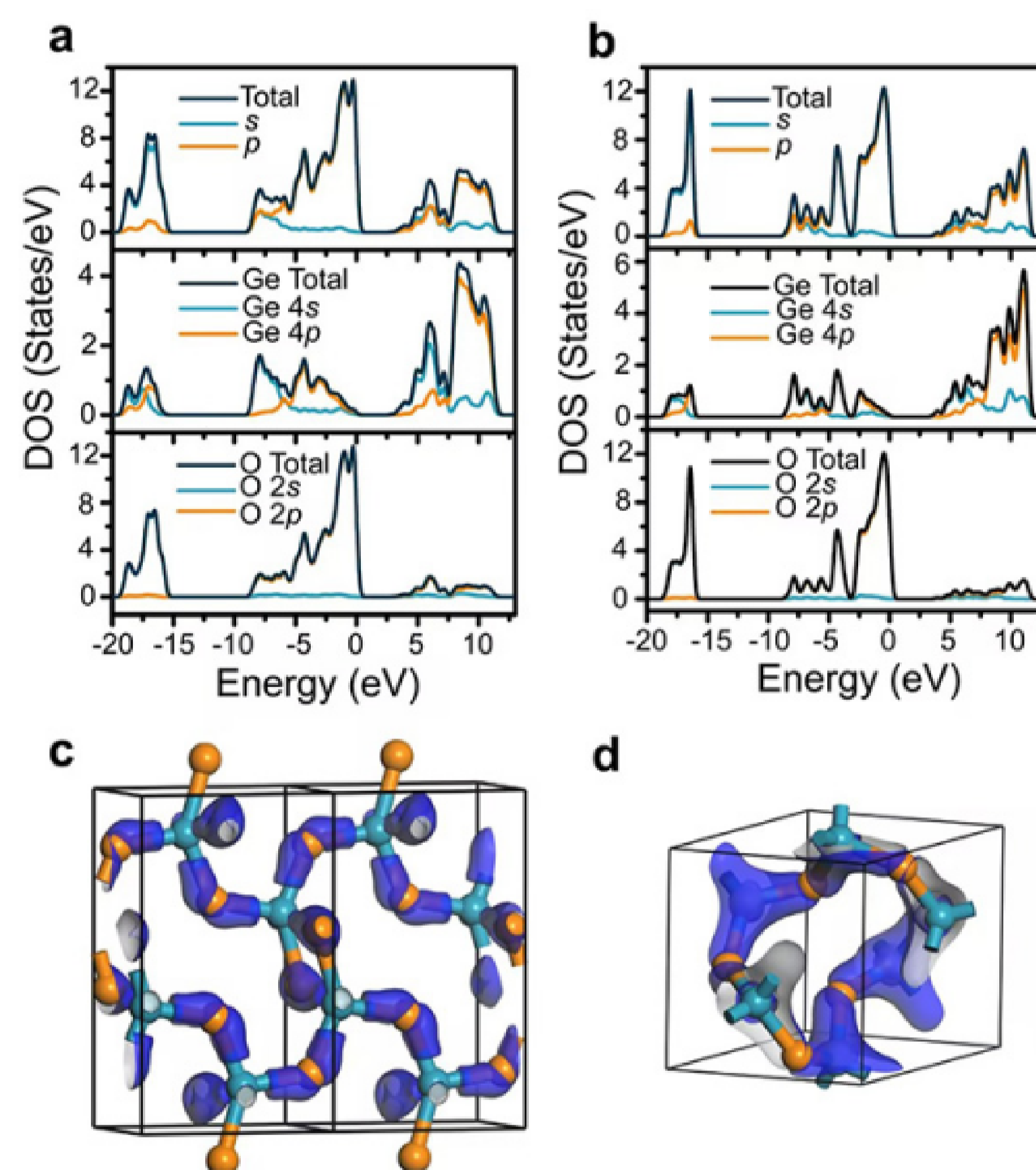
图2. \text{GeO}_2 熔体中两种聚合物 ( [\text{GeO}_2]_n 链和 [\text{GeO}_4]_n 网络) 的电子结构。(a) [\text{GeO}_2]_n 链的总态密度和分态密度；(b) [\text{GeO}_4]_n 的总态密度和分态密度；(c) [\text{GeO}_2]_n 在-8.0到-7.1 eV能量区间的成键轨道；(d) [\text{GeO}_4]_n 在-8.6到-7.5 eV能量区间的成键轨道。
