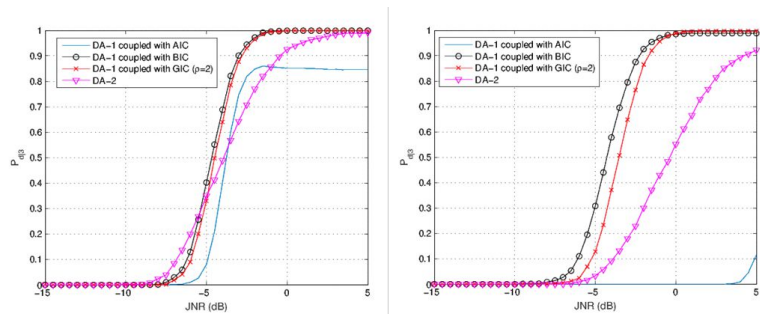
图2 检测性能：左N=16, K=18；右N=16, K=14
