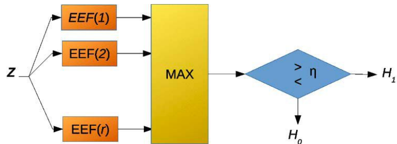
图1 MLRT方法结构框图
