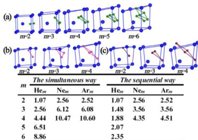
图2. 钨中热负荷缓冲剂杂质 (氢、氦、氩) 间隙团簇稳定构型和相应结合能
