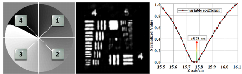
图1 涡旋光的相移干涉区域(左), 分辨率板的重构像(中)及自动对焦曲线(右)
