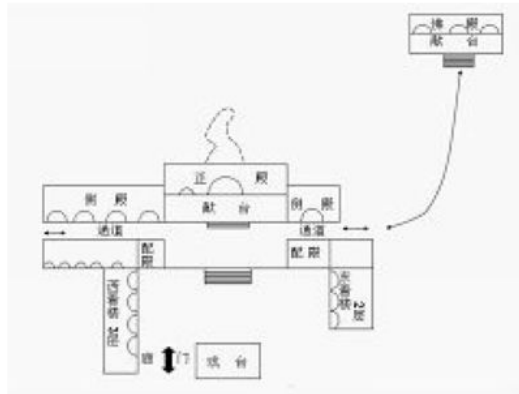
图1: 五龙洞圣母庙平面示意图
